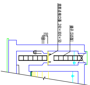
A' - A' 断面图 S=1/50
