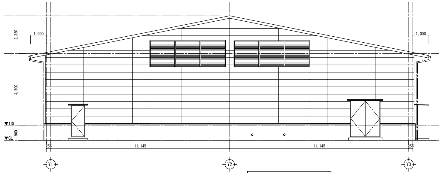
北面 立面图 S:1/100
