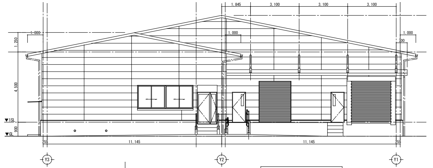
南面 立面图 S:1/100
