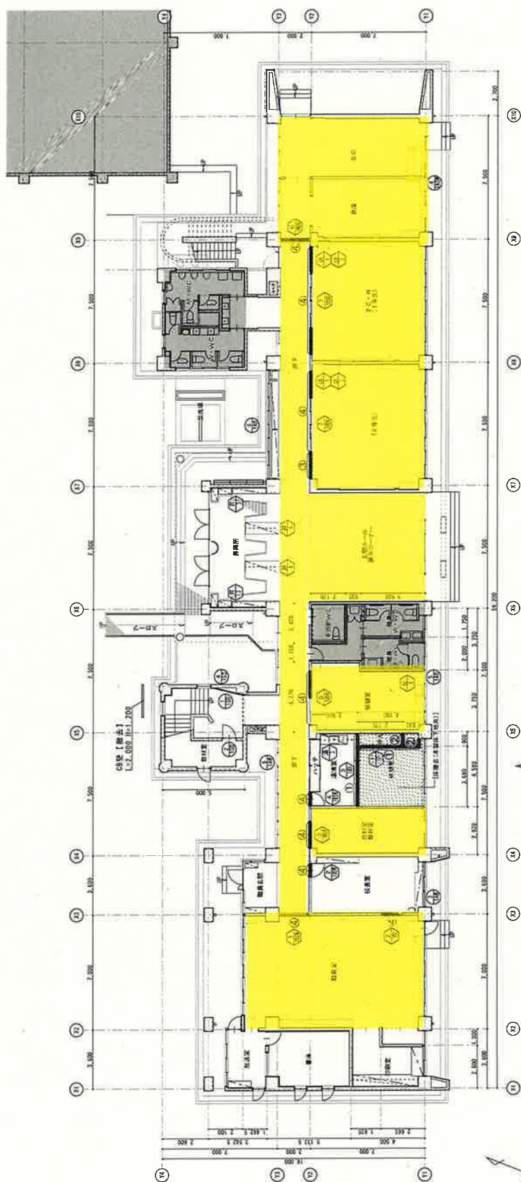
【図四】校舎棟 1 階平面図 S=1:150
