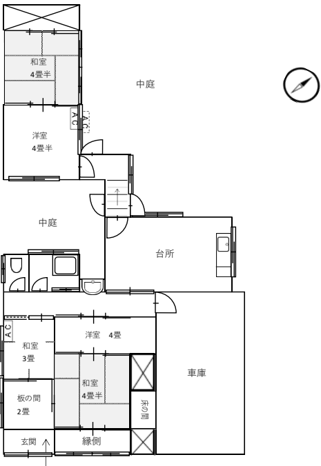
【間取り図】
