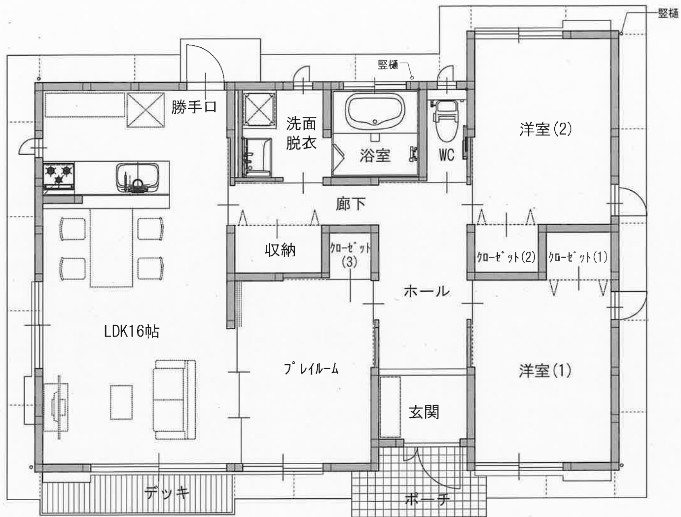
1号棟 平面図
