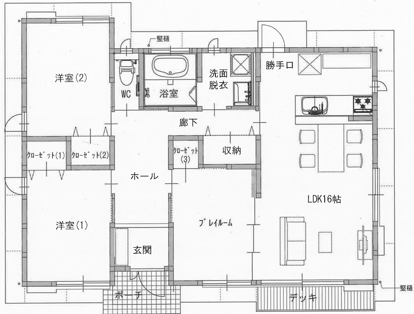
3号棟 平面図
