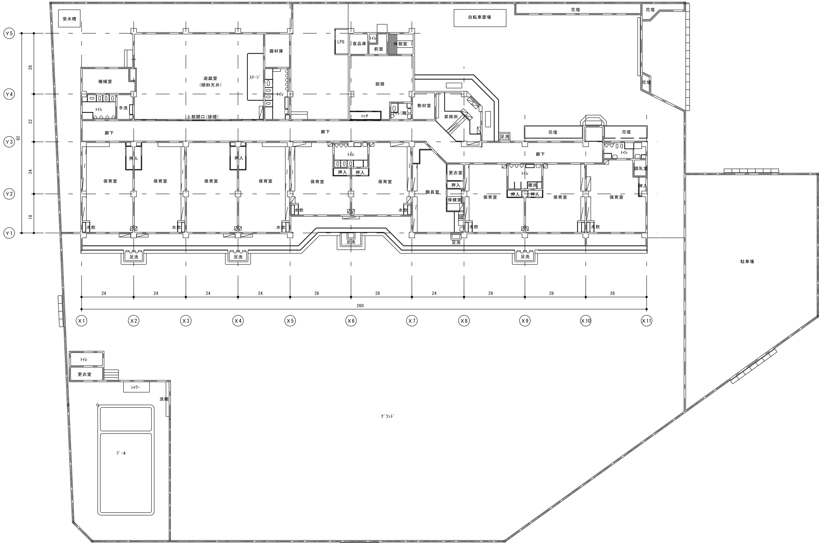
配置図 S=1:250
