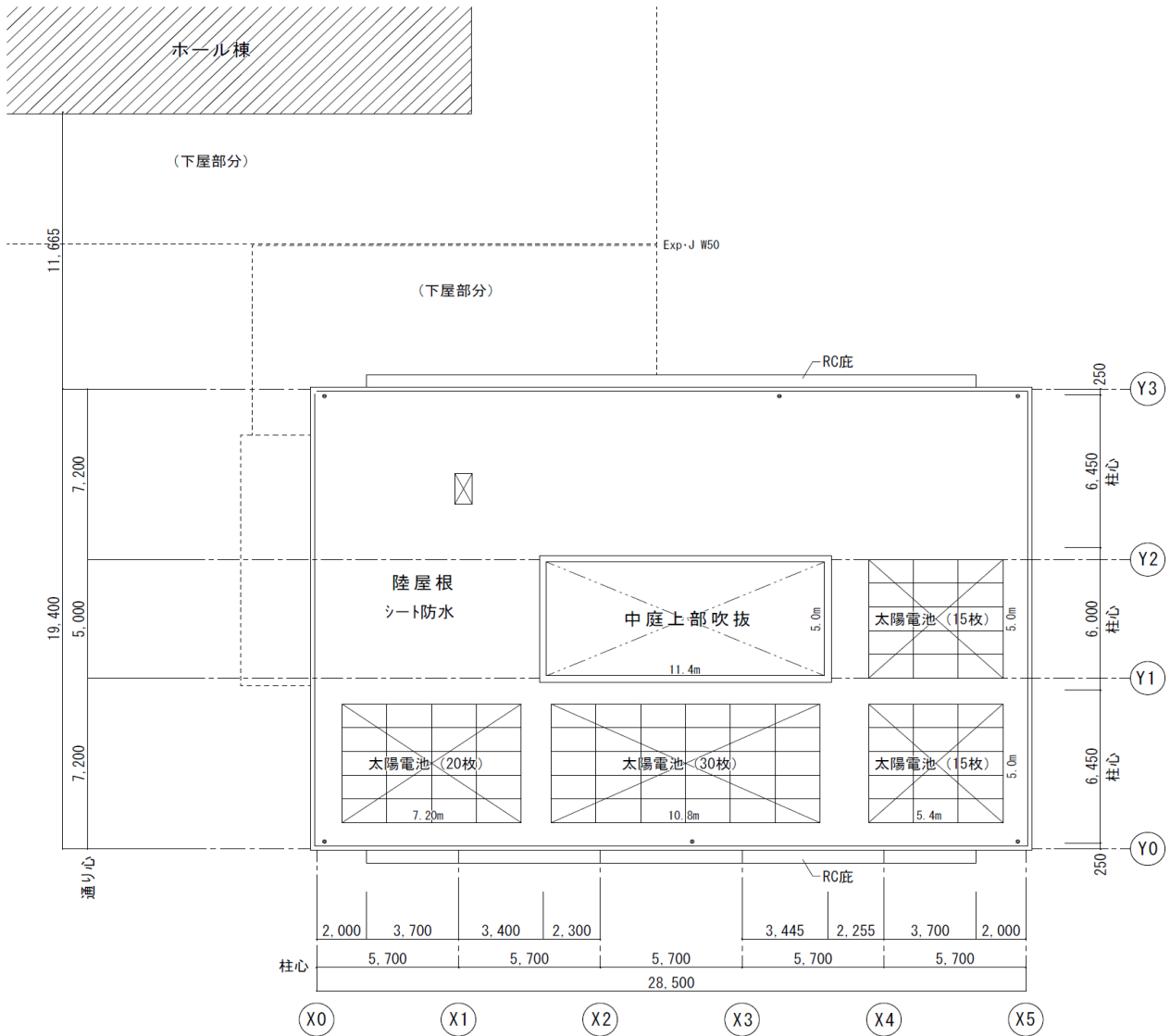
屋根伏図 S=1:250
