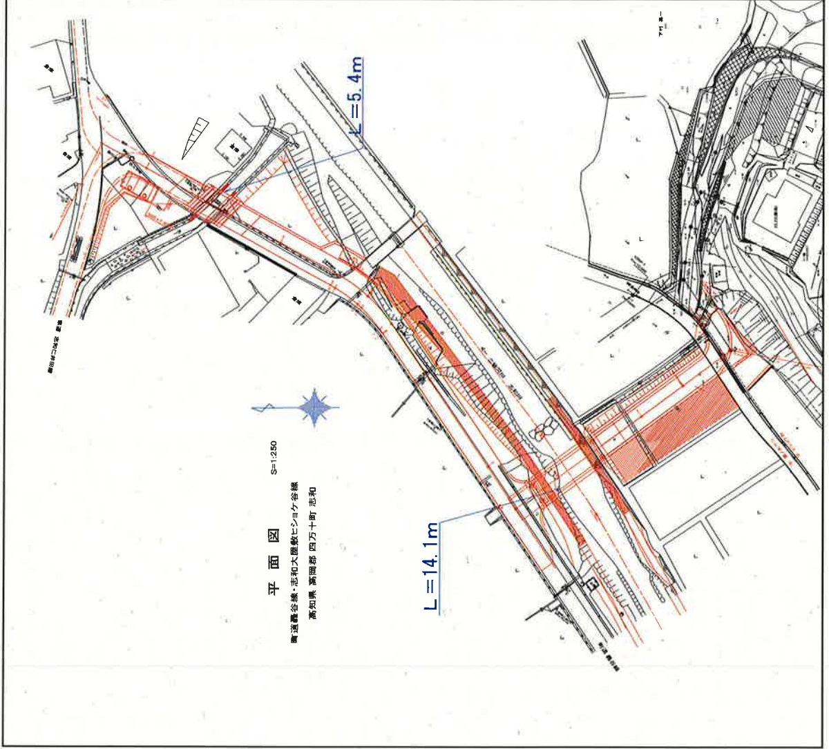
町道計画平面図
